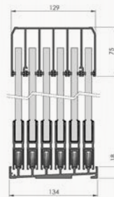
Afmetingen 6-sporige rails, verkrijgbaar in de lengte: 5900mm.
