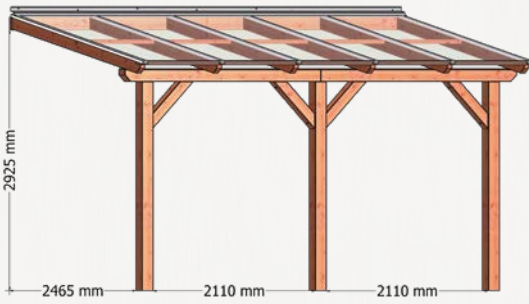
Terrasoverkapping La Véranda 5000x3000mm
