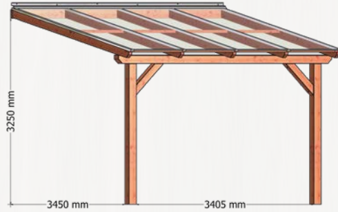
Terrasoverkapping La Véranda 4000x4000mm
