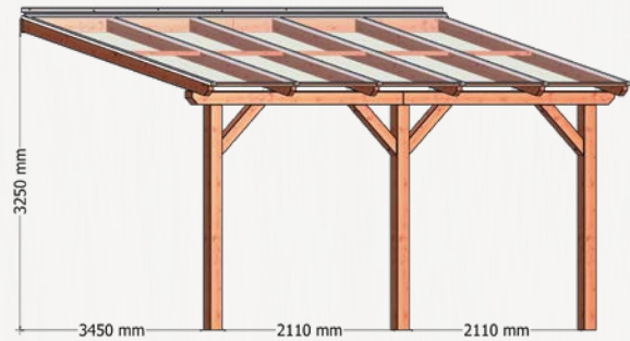
Terrasoverkapping La Véranda 5000x4000mm
