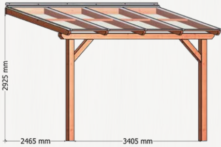
Terrasoverkapping La Véranda 4000x3000mm
