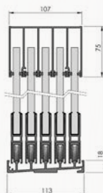
Afmetingen 5-sporige rails, verkrijgbaar in de lengte: 4900mm.
